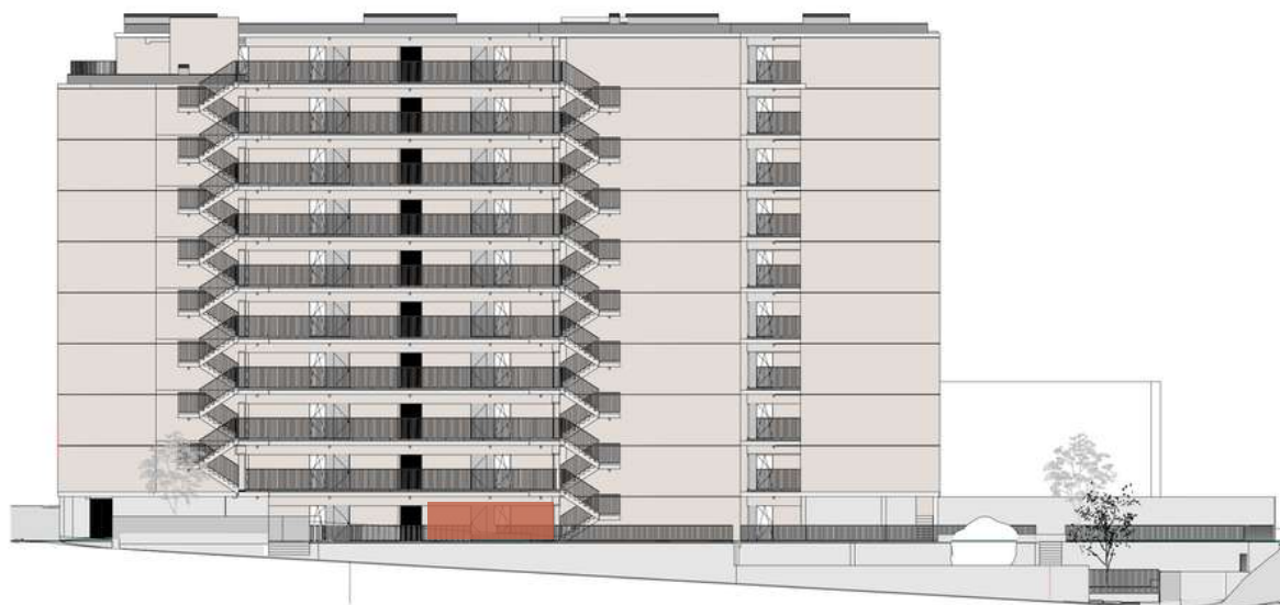
ALÇADO PRINCIPAL
